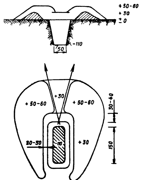
Одиночный окоп для стрельбы из автомата стоя
